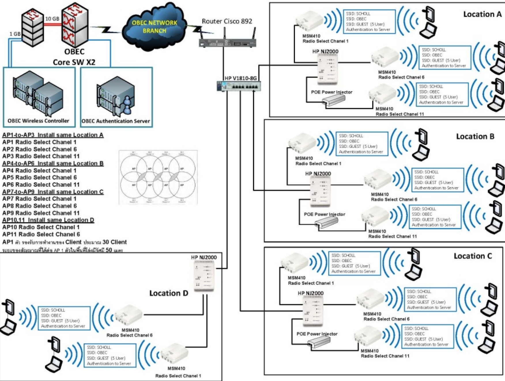
ตัวอย่างการออกแบบติดตั้งอุปกรณ์ “โครงการพัฒนาระบบเครือข่ายไร้สายสำหรับสถานศึกษาในสังกัด สพฐ.” ปีงบประมาณ 2555
