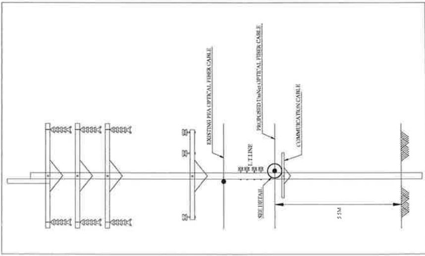
รูปแบบการติดตั้งสายเคเบิลใยแก้วนำแสง ADSS 24 F
