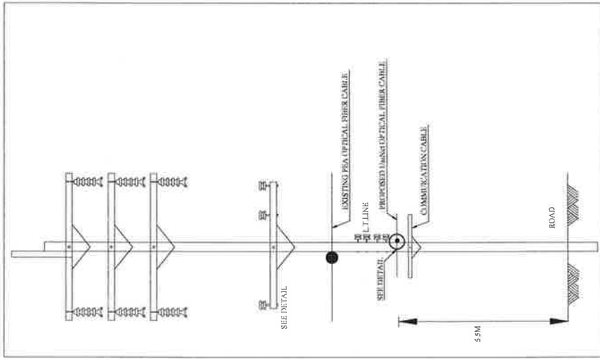
รูปแบบการติดตั้งสายเคเบิลใยแก้วนำแสง DROP WIRE 12F บนเสาการไฟฟ้าส่วนภูมิภาค ขนาด 115 KV
